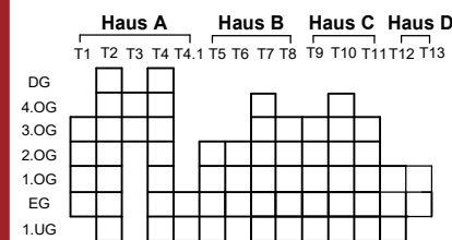
Treppenschnitt
